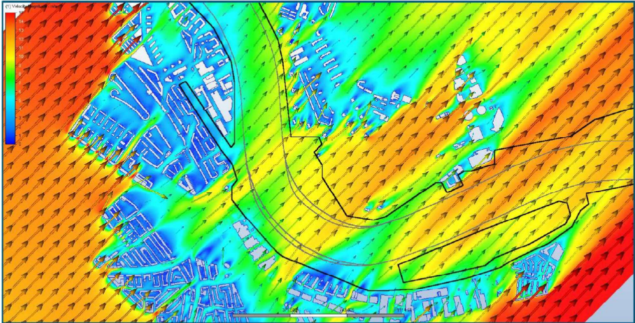
Figuur 4-13 Huidige situatie ZW wind op 6 m hoogte
