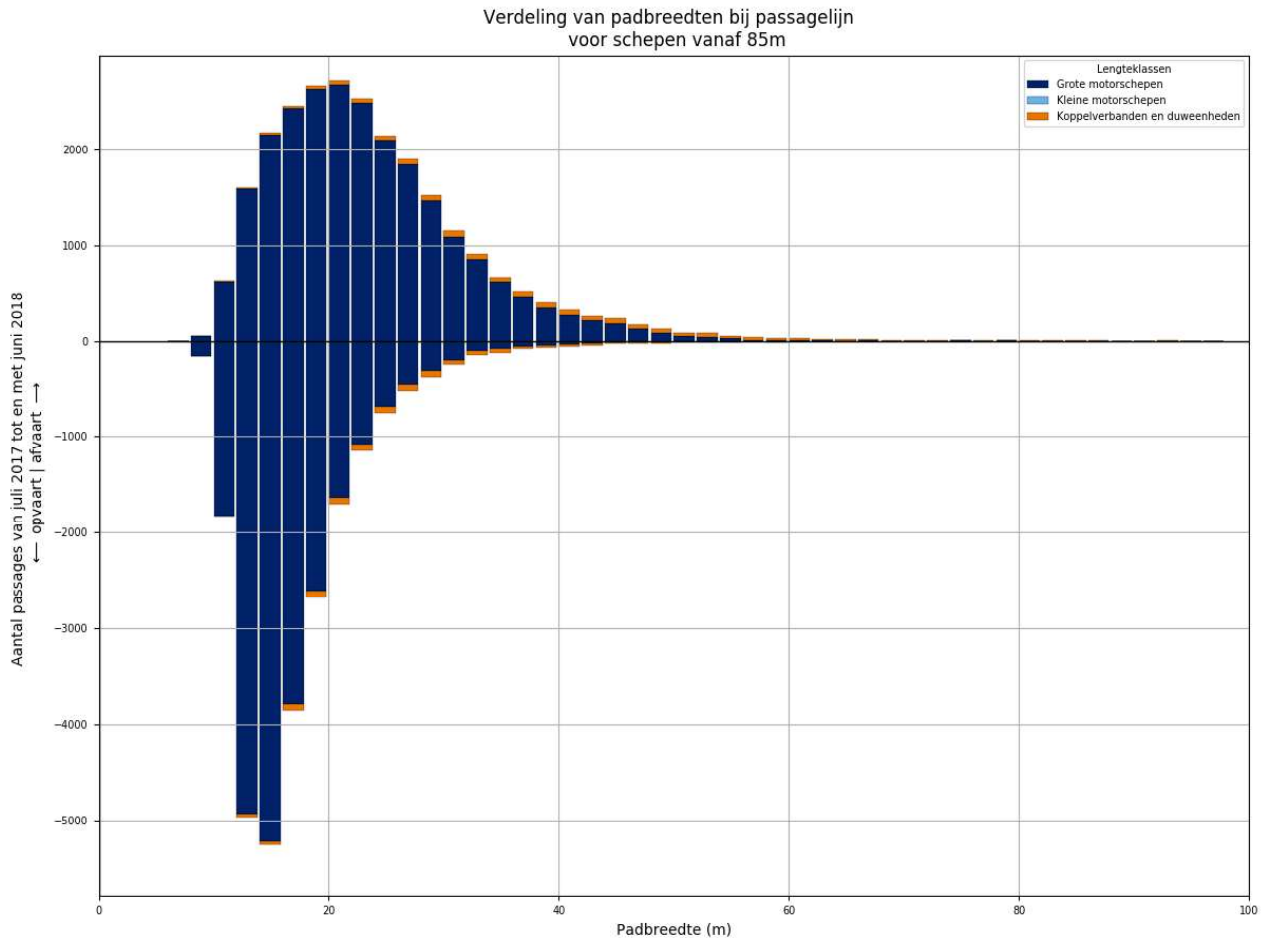
Figuur 3-4 Padbreedte van schepen vanaf 85 m
