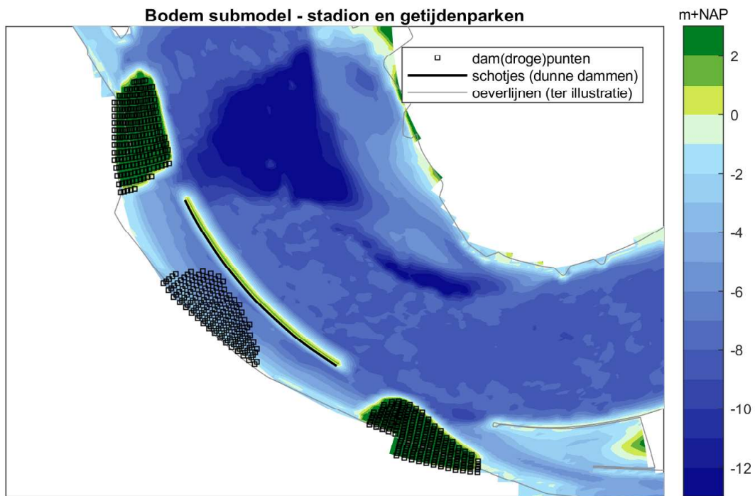
Figuur 4-3 Bodemligging met diep gedeelte aan benedenstreamse kant van bocht
