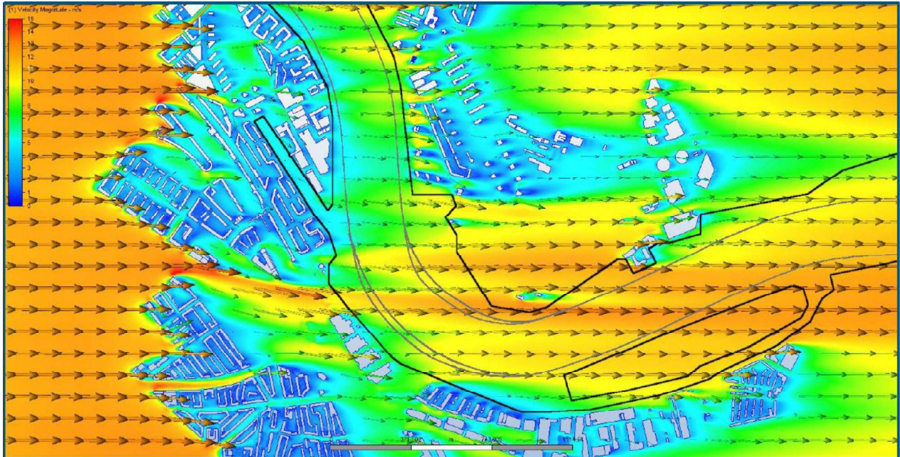
Figuur 4-15 Huidige situatie W wind op 6 m hoogte
