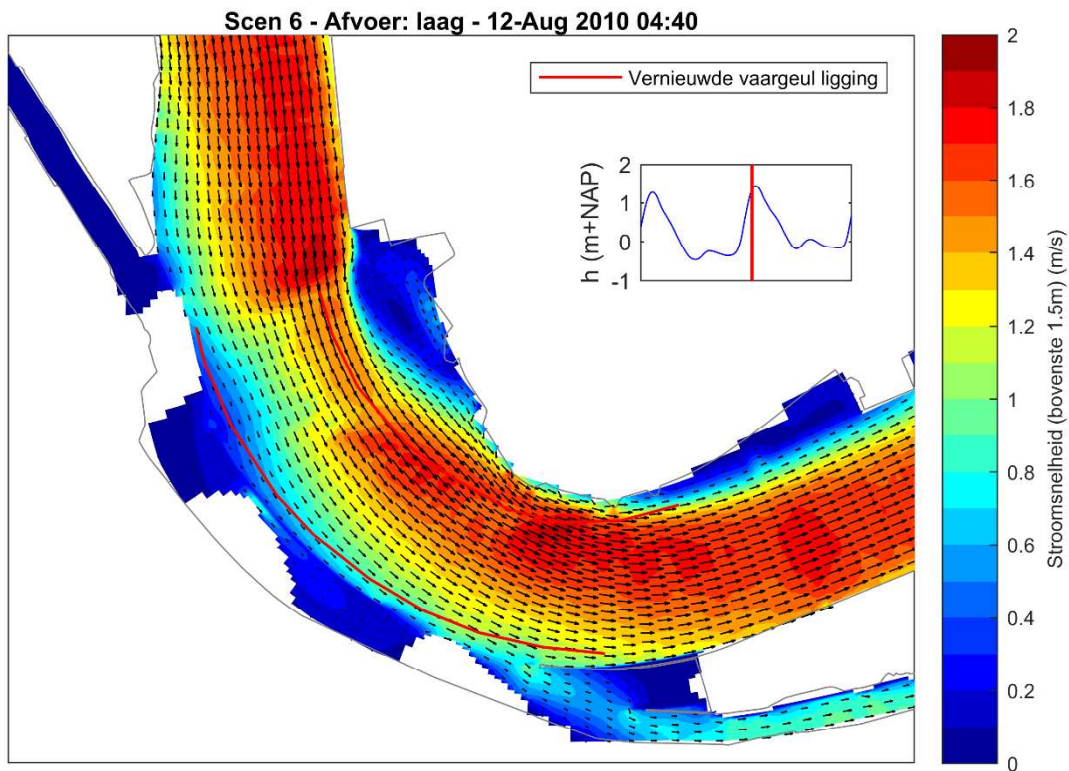
Figuur 4-9 Stroomsnelheden scen 6 (max. vloed) voor bovenste 1,5 m laag
