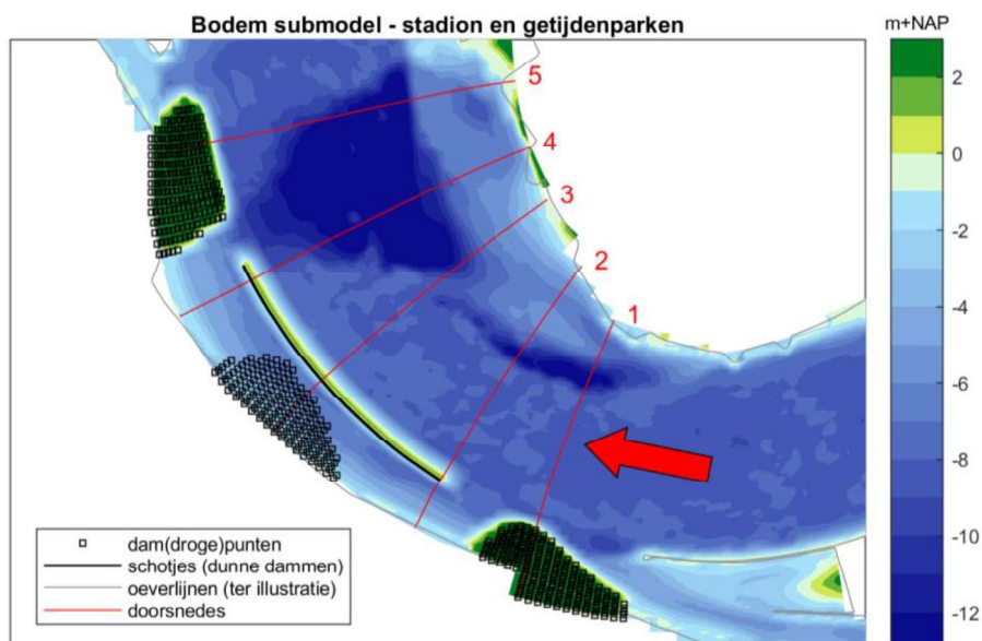
Figuur 3.1: Locaties van de dwarsdoorsnedes. De rode pijl weergeeft de richting vanaf welke de dwarsdoorsnedes worden bekeken.
