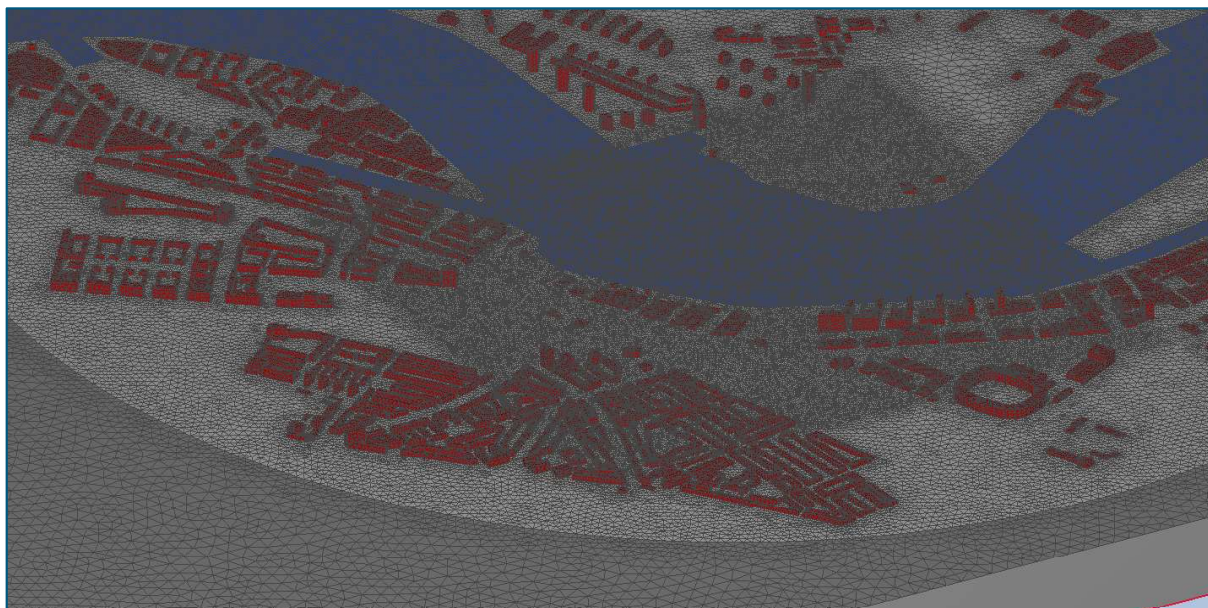
Afbeelding 3-1: Overzicht rekenrooster
